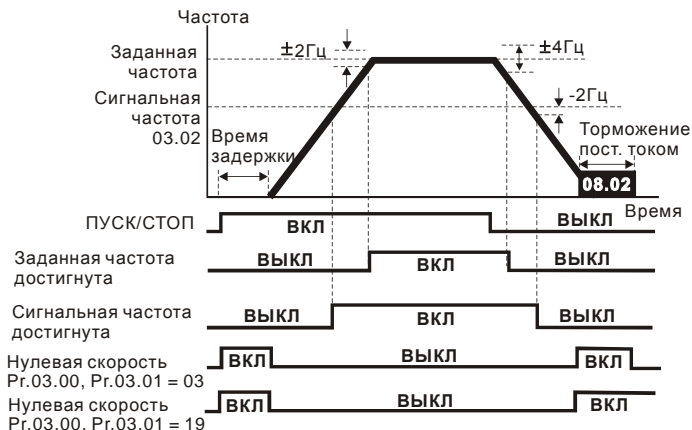
Диаграмма работы дискретных выходов при сигнализации достижения частоты и нулевой скорости
