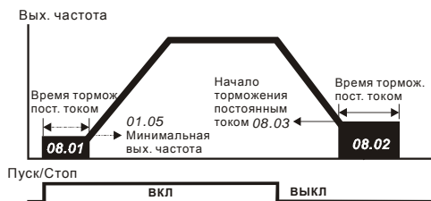
Торможение постоянным током
